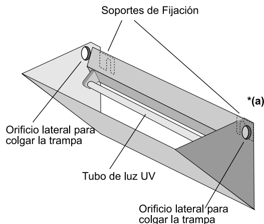
Figura 1: Instalación del equipo en la pared.
